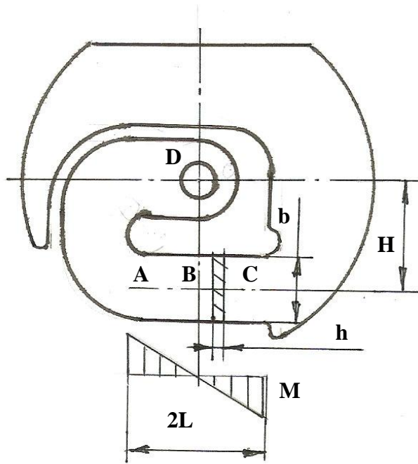
图 2 平板式半环形支撑悬臂梁弹性元件
