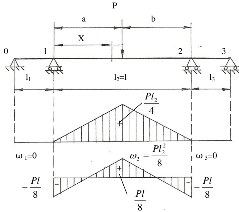
图 3 中心应变梁计算模型、载荷面积图和弯矩图
