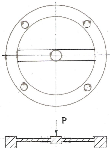
图 1 平板式双端固支梁弹性元件及电阻应变计粘贴位置
