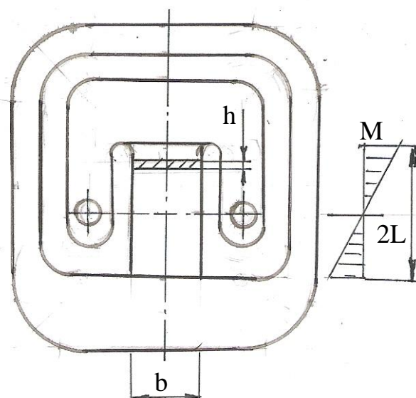
图 2 平板式环形支撑悬臂梁弹性元件
