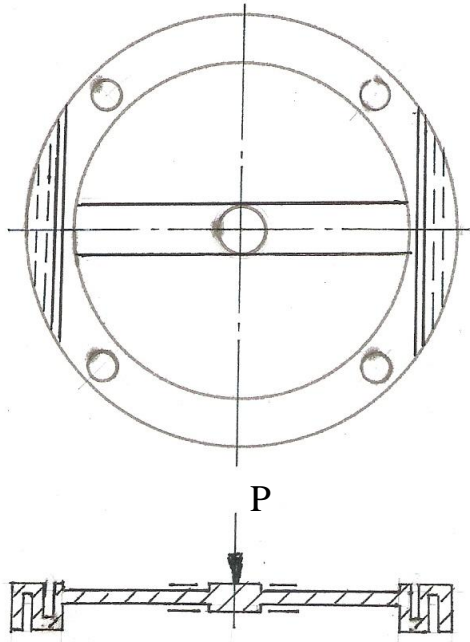
图 4 应变梁支座开槽位置及方向图
