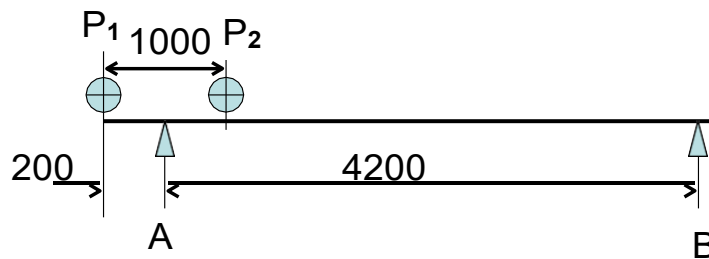
图 5 T6 检衡车载荷示意图
