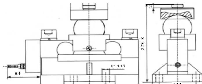
图 3 桥式称重传感器示意图
