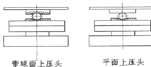
图 6 多只称重传感器压头示意图
