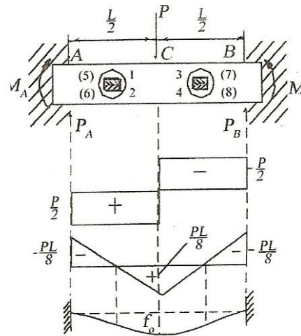
图 4 桥式称重传感器受力示意图
