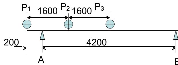
图 1 机车主动轴载荷示意图
