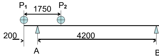
图 2 转向架载荷示意图
