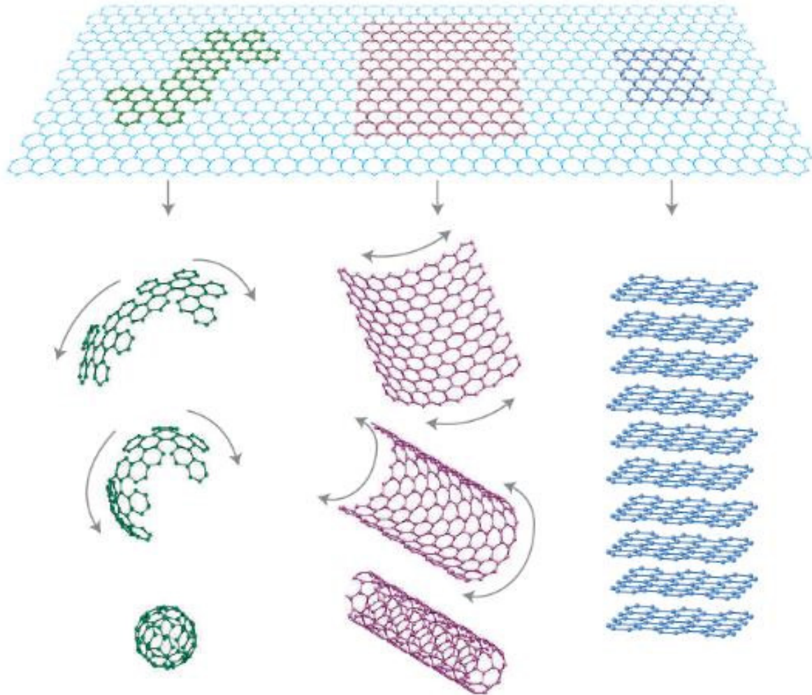
图 石墨烯是构成富勒烯（左）、碳纳米管（中）和石墨（右）的基础材料 [3]
